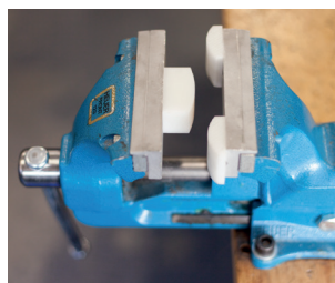
Afbeelding 4: Driepuntsbuigmal
